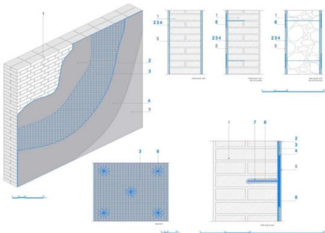
Slika 81 Detalji izvedbe ojačanja FRCM sustavom - redosljed izvođenja sustava
