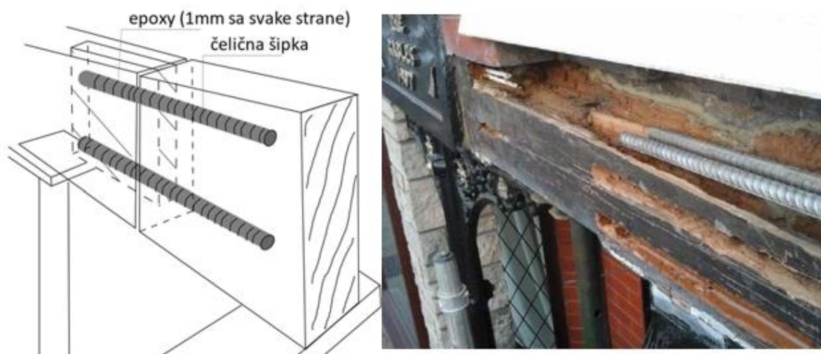
Slika 93: Sanacija drvenih greda čeličnim šipkama i epoksidnim mortom
