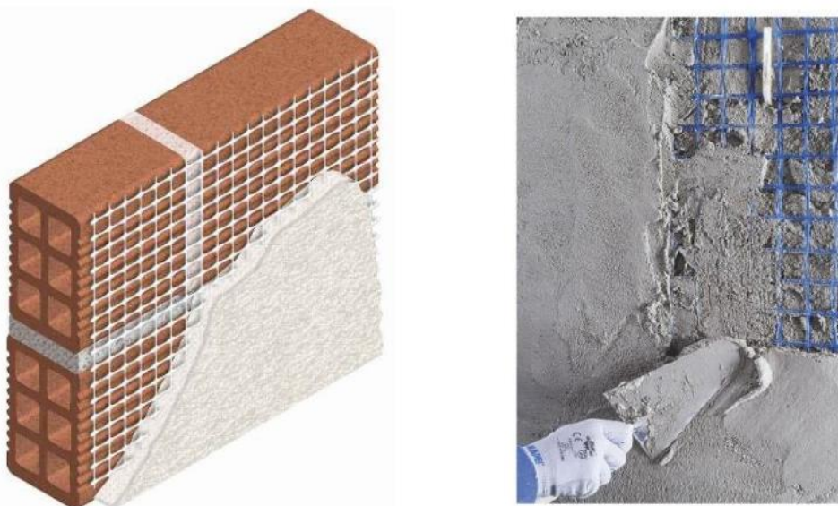
Slika 79 Detalji izvedbe ojačanja FRCM sustavom
