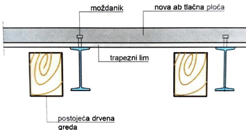
Slika 91: Presjek AB tlačne ploče
