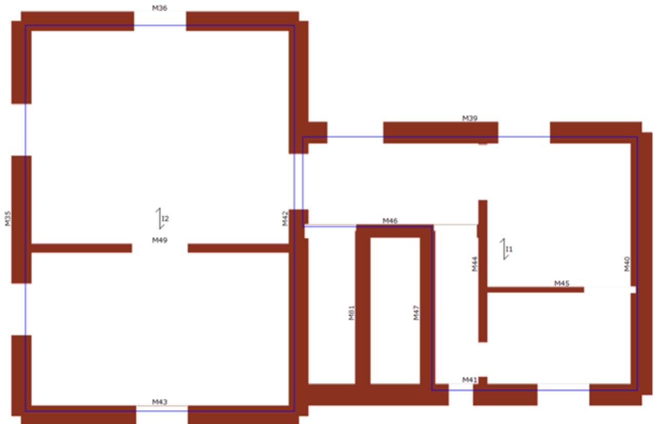
Slika 99 Tlocrt 1. kata modela
