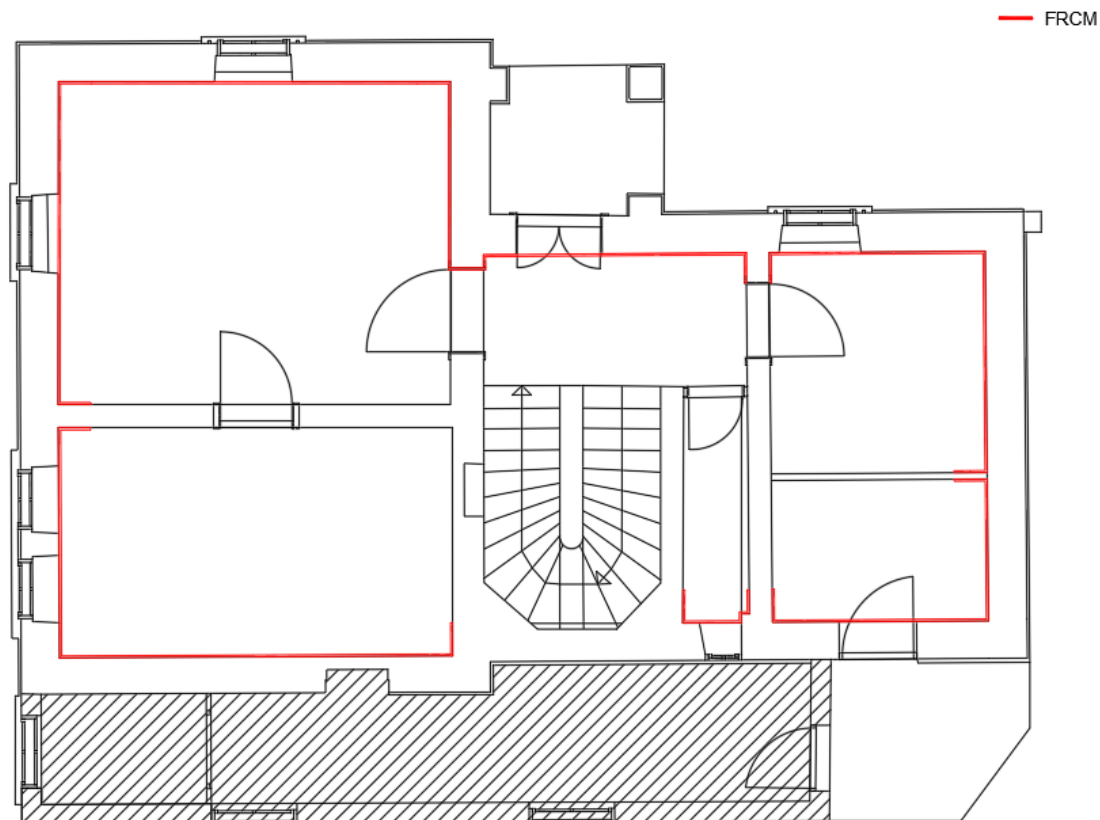
Slika 84: Prizemlje – lokacije FRCM sustava za ojačanje zidova
