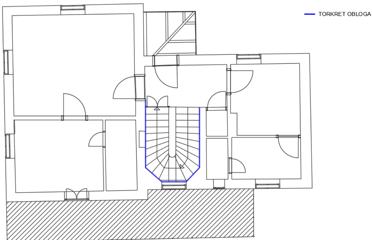
Slika 90: 1. kat – lokacije torkret obloge za ojačanje zidova
