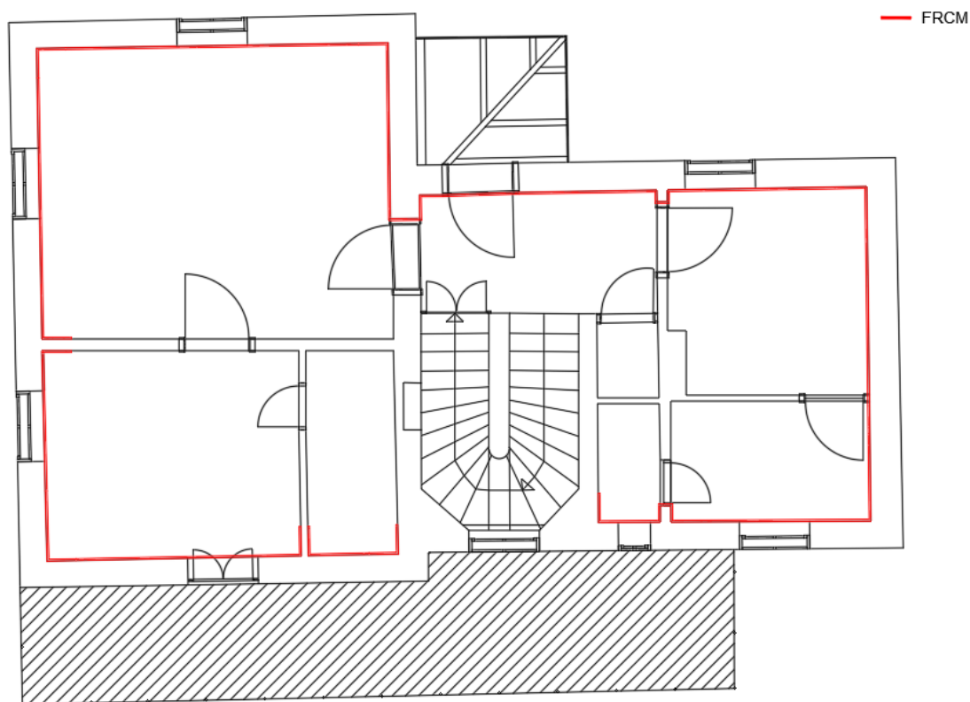
Slika 85: 1. kat – lokacije FRCM sustava za ojačanje zidova
