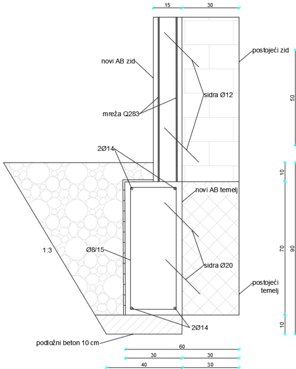
Slika 97: Prikaz ojačanja zida novim AB zidom
