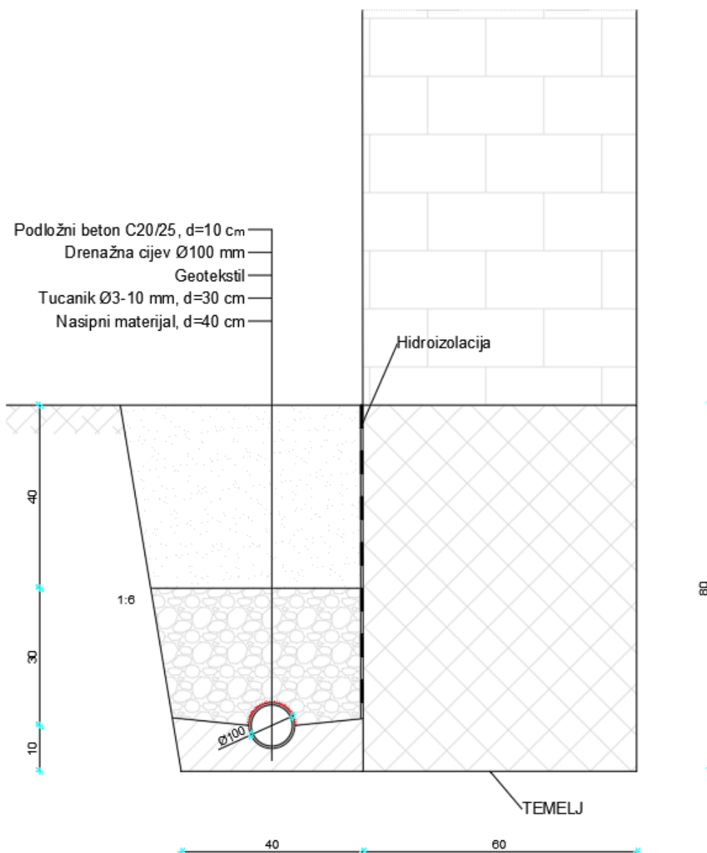
Slika 96: Prikaz izvedbe drenažnog sustava
