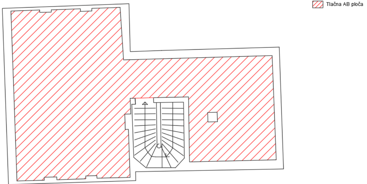
Slika 92: Tlocrt potkrovlja - lokacije izvedbe AB tlačne ploče
