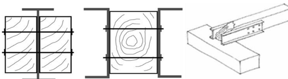
Slika 94: Sanacija i pojačanje drvenih elemenata dodavanjem čeličnih elemenata
